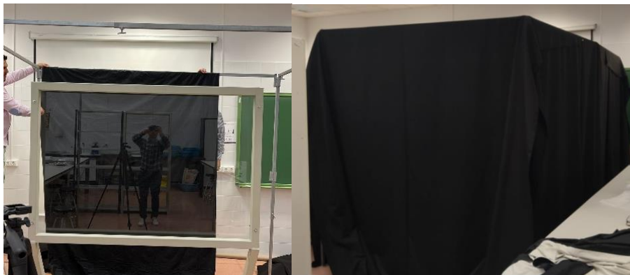
Fig. 5. Colocación de estructura de cerramiento y cubrimiento del Lightboard studio.
